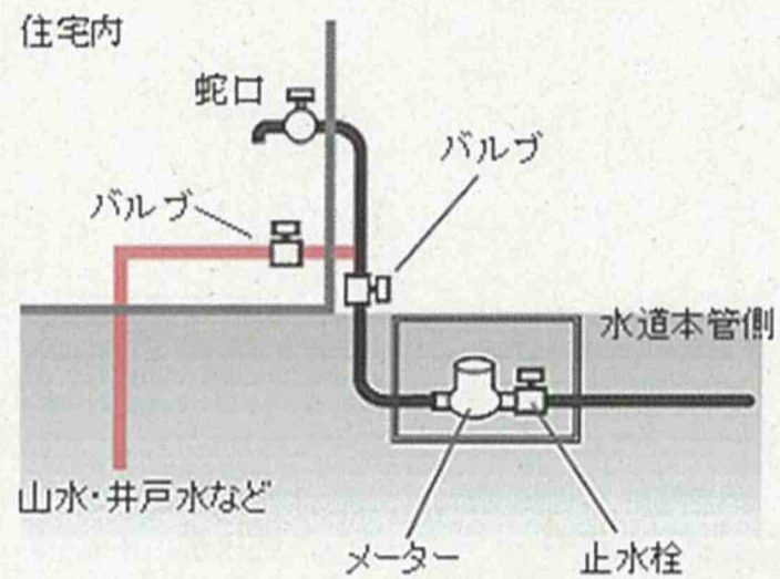
【クロスコネクションの例】
