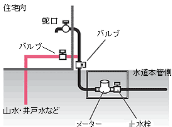
【クロスコネクションの例】
