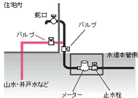
【クロスコネクションの例】
