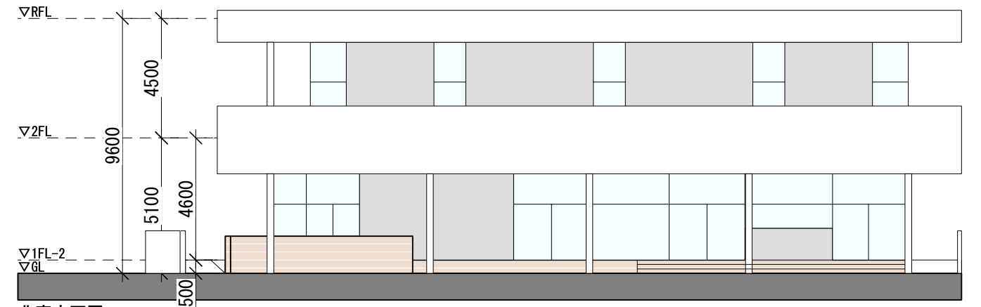
北東立面図
