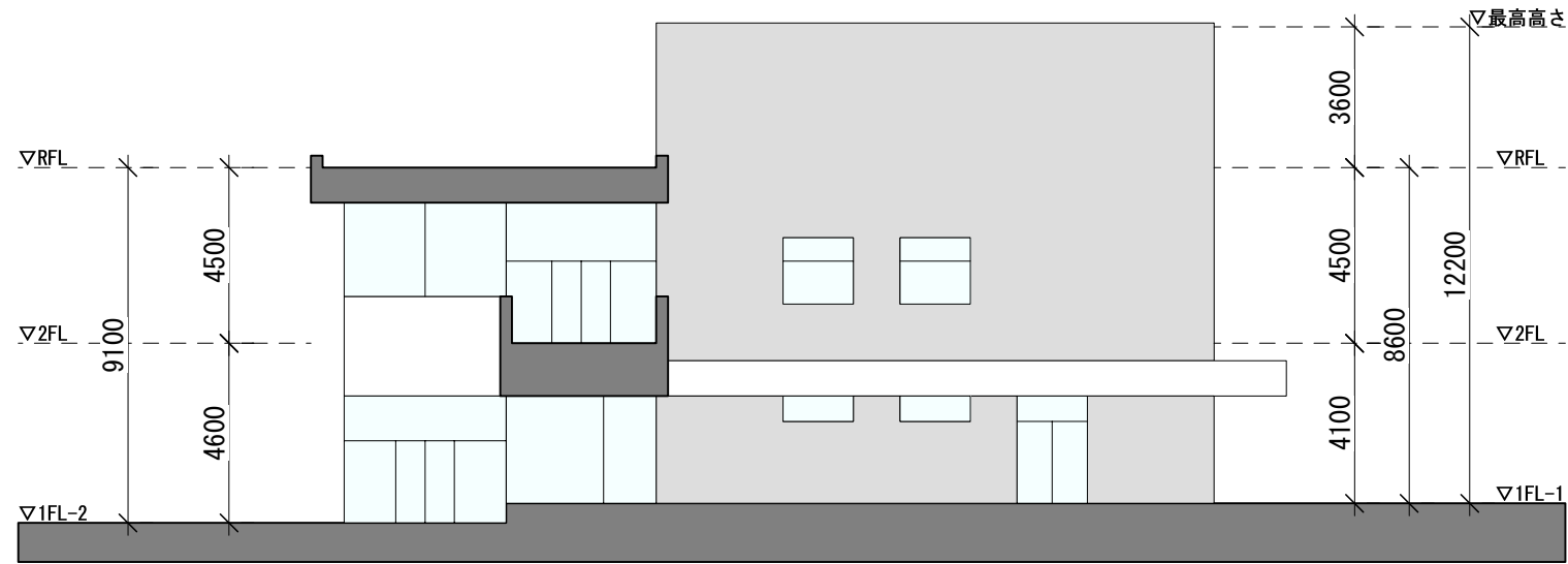
南西立面図
